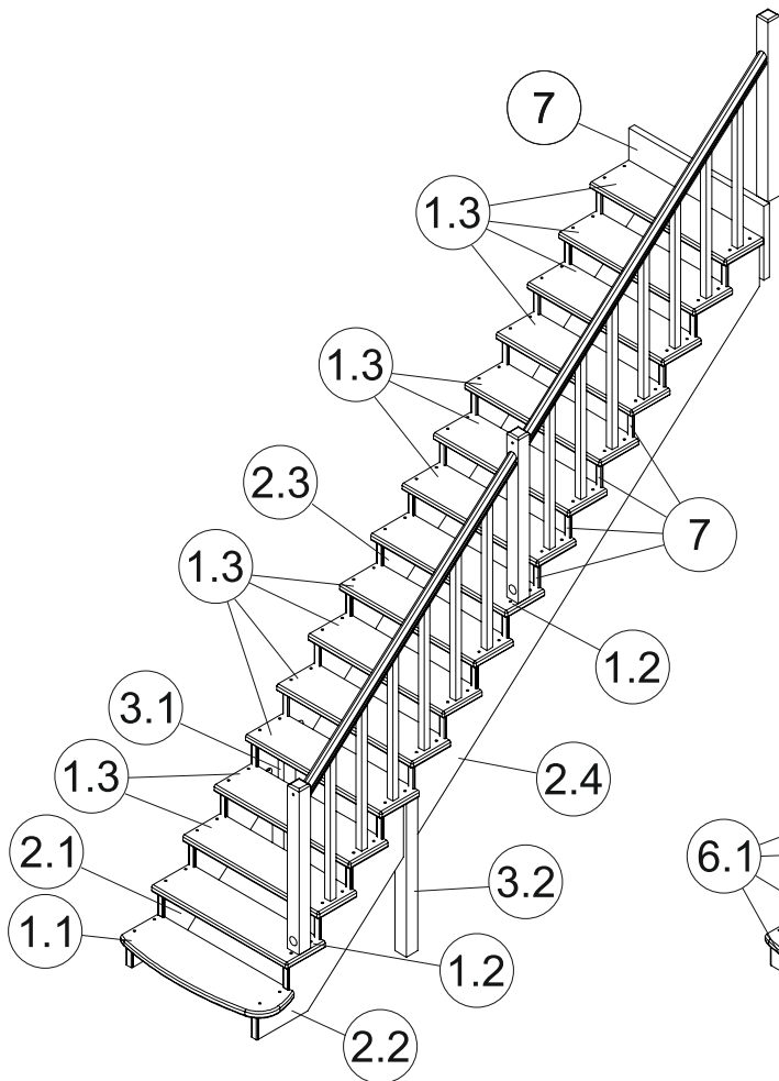
Без подступенников
