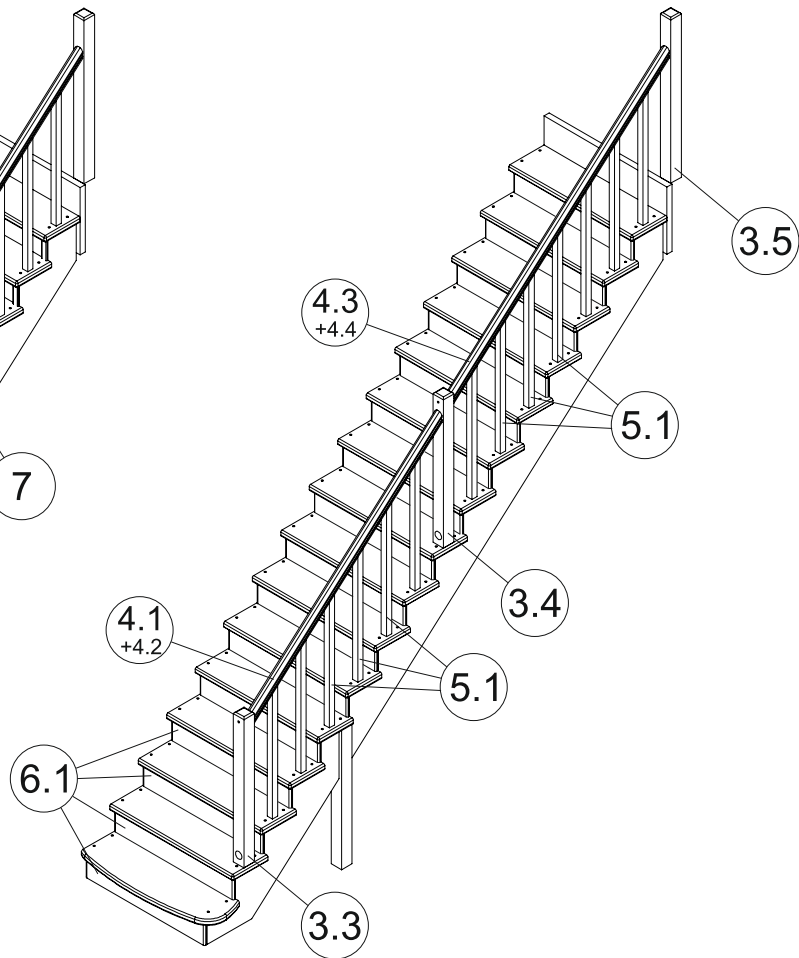
С подступенниками
